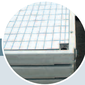
Massivbalkon mit Belag und Aussparung für Wasserablauf.
