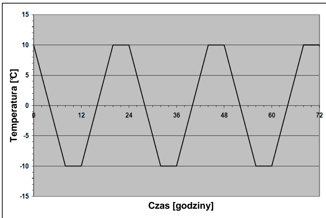
Rys.1 Wykres profilu temperatury w teście zamrażania-rozmrażania
