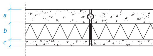
Horizontalsnitt – väggskarv
