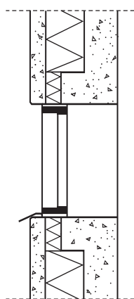
Vertikalsnitt – fönstersmyg
