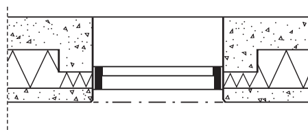
Horizontalsnitt – fönstersmyg
