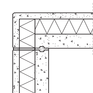
Horizontalsnitt – ytterhörn
