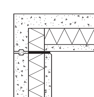
Horizontalsnitt – innerhörn
