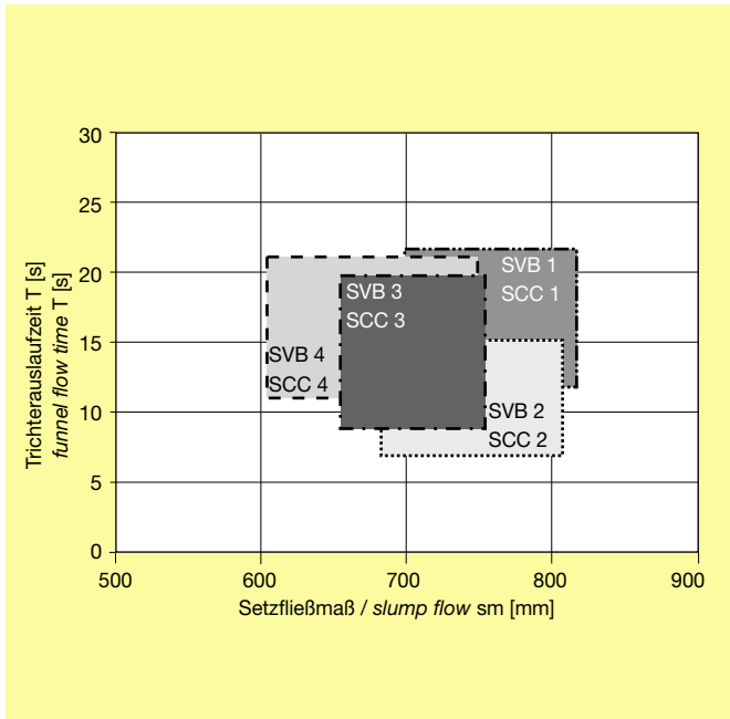
Bild 3: Verarbeitbarkeitfenster für vier verschiedene SVB [6]
