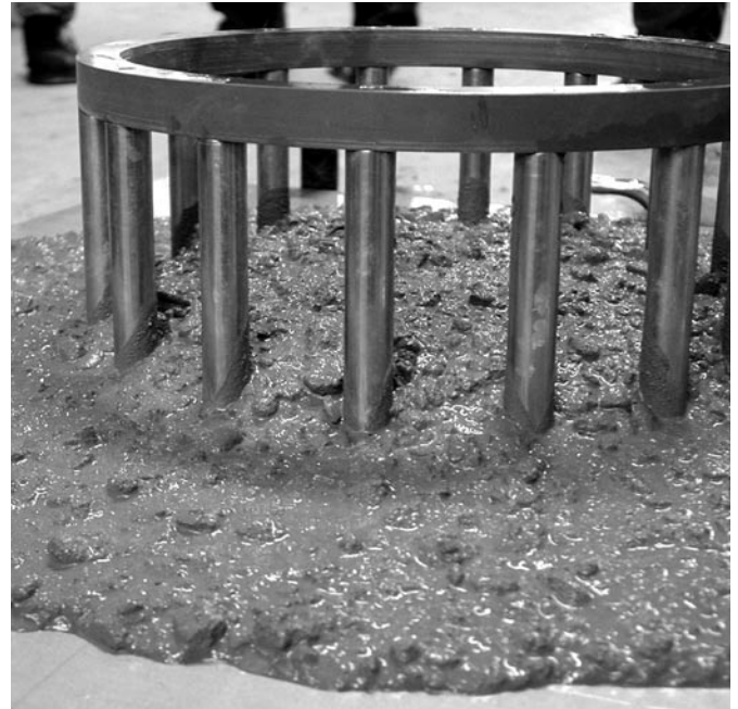
Bild 1: Ermittlung des s_{m_b} -Wertes
